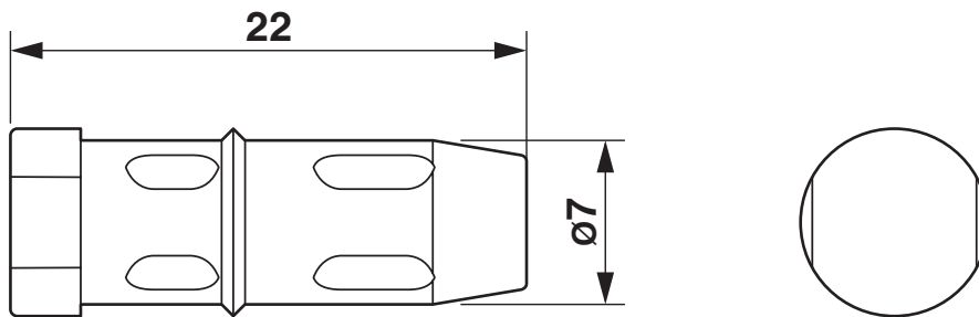
Rysunek wymiarowy
