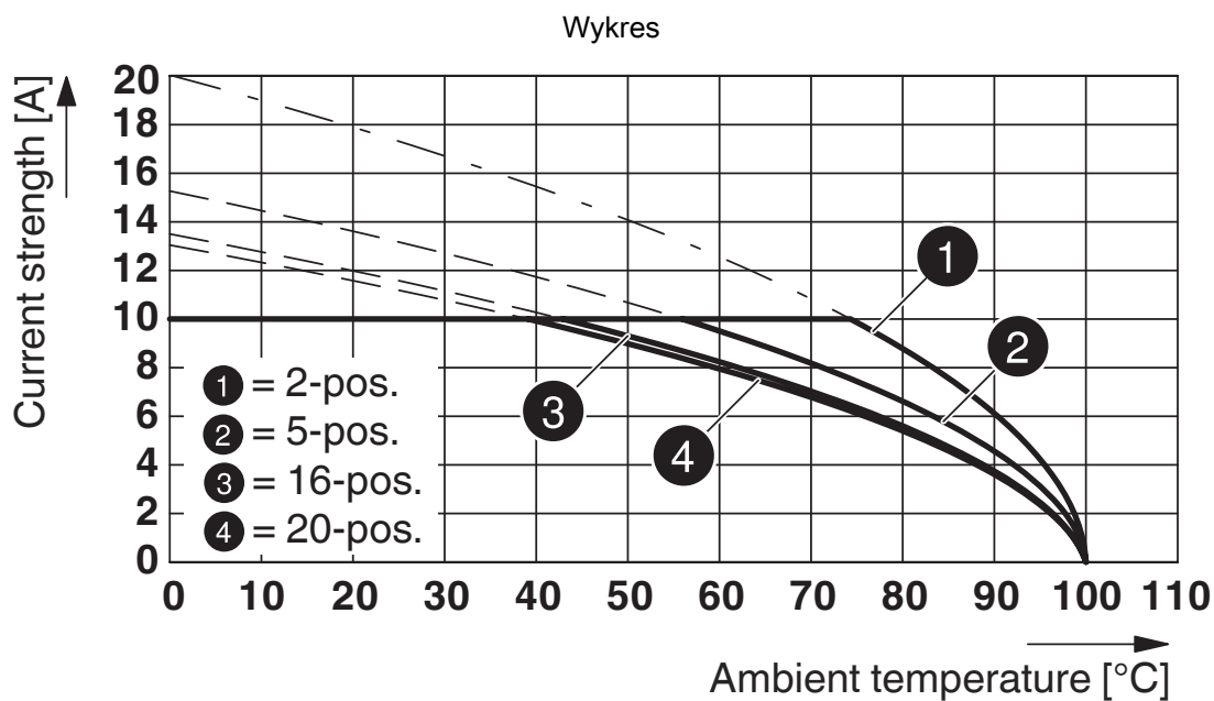
Typ: SMSTB 2,5/...-ST-5,08 z MDSTB 2,5/...-G1-5,08
