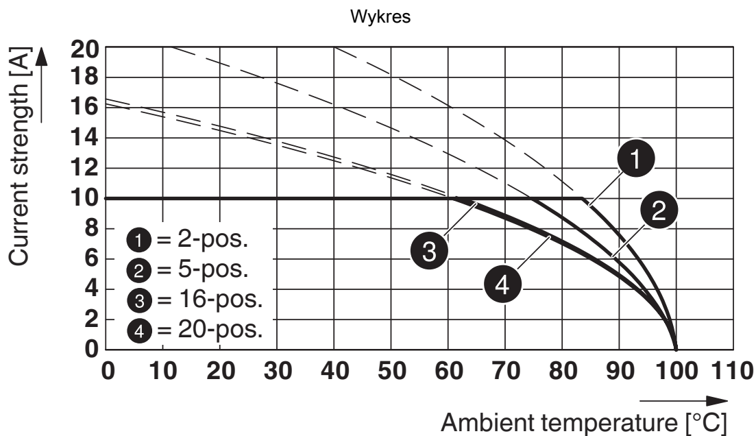
Typ: FKCS 2,5/...-ST-5,08 z MDSTB 2,5/...-G1-5,08
