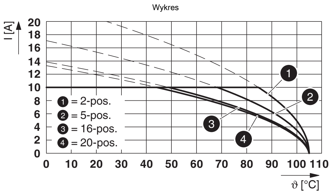
Typ: IC 2,5/...-G-5,08 z MDSTB 2,5/...-G1-5,08
