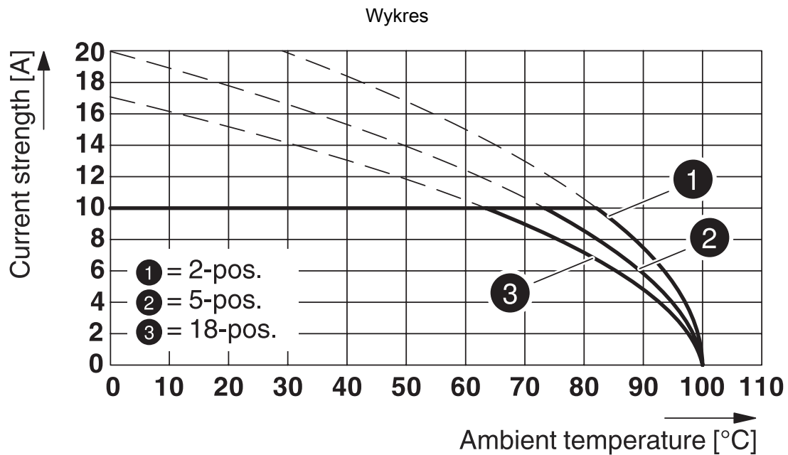
Typ: FKCN 2,5/...-ST-5,08 z MDSTB 2,5/...-G1-5,08
