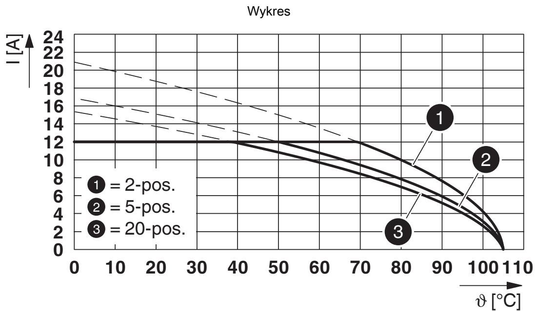
Typ: FKCT 2,5/...-ST-5,08 z MSTBV 2,5/...-G-5,08
