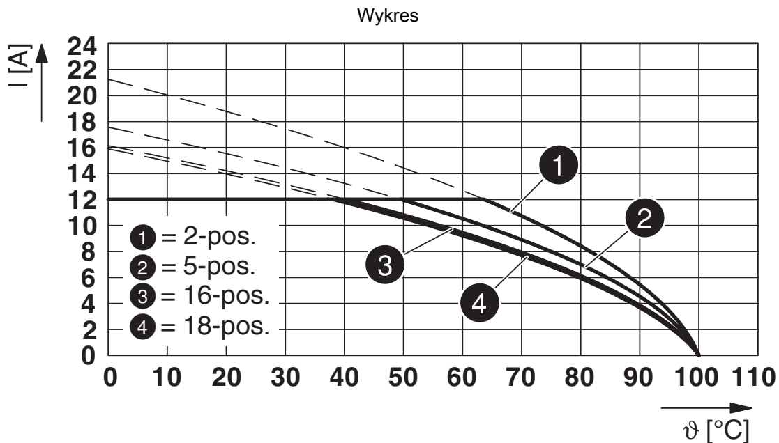
Typ: FKCV(W/R) 2,5/...-ST z MSTBV 2,5/...-G
