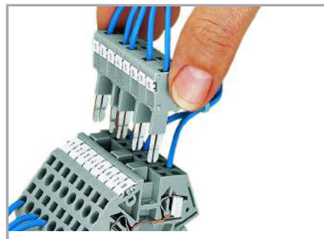
Moduły pomiarowe typu B z zaciskiem CAGE CLAMP®
