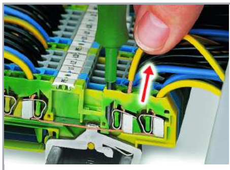
Zacisk CAGE CLAMP®
