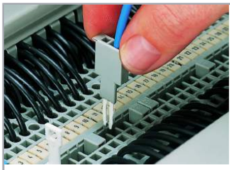
Pomiar za pomocą wtyku pomiarowego Wtyk pomiarowy z zaciskiem CAGE CLAMP®
