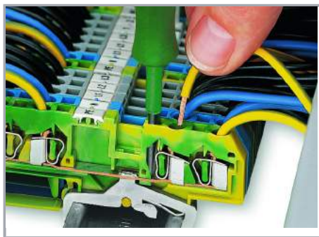
Zacisk CAGE CLAMP®
