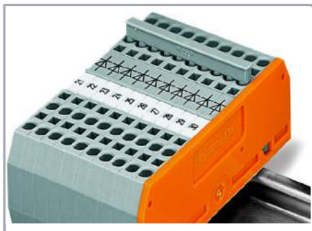
Mostkowanie przy użyciu grzebieni mostkujących Grzebień mostkujące wciskać do oporu!
