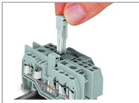
Mostkowanie złączki do większych przekrojów ze złączką do mniejszych przekrojów przy pomocy mostków redukcyjnych
