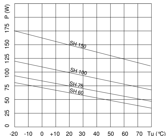
Leistung in Abhängigkeit von der Umgebungstemperatur / Thermal output depending upon ambient temperatur
