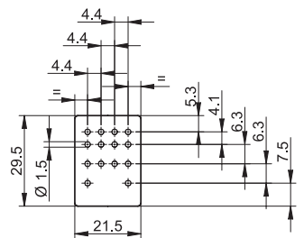
Rysunek otworów montażowych
