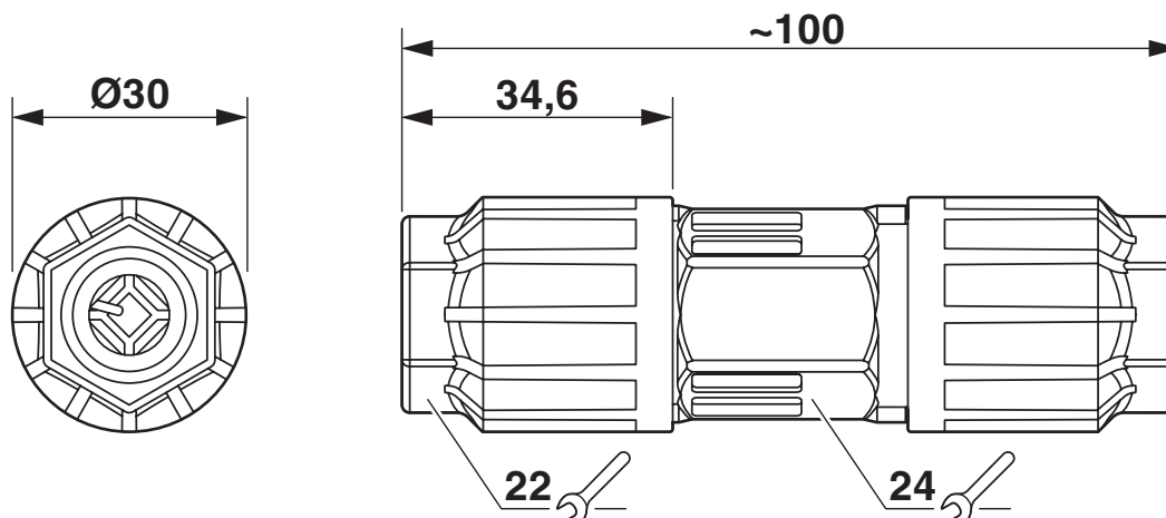
Rysunek wymiarowy
