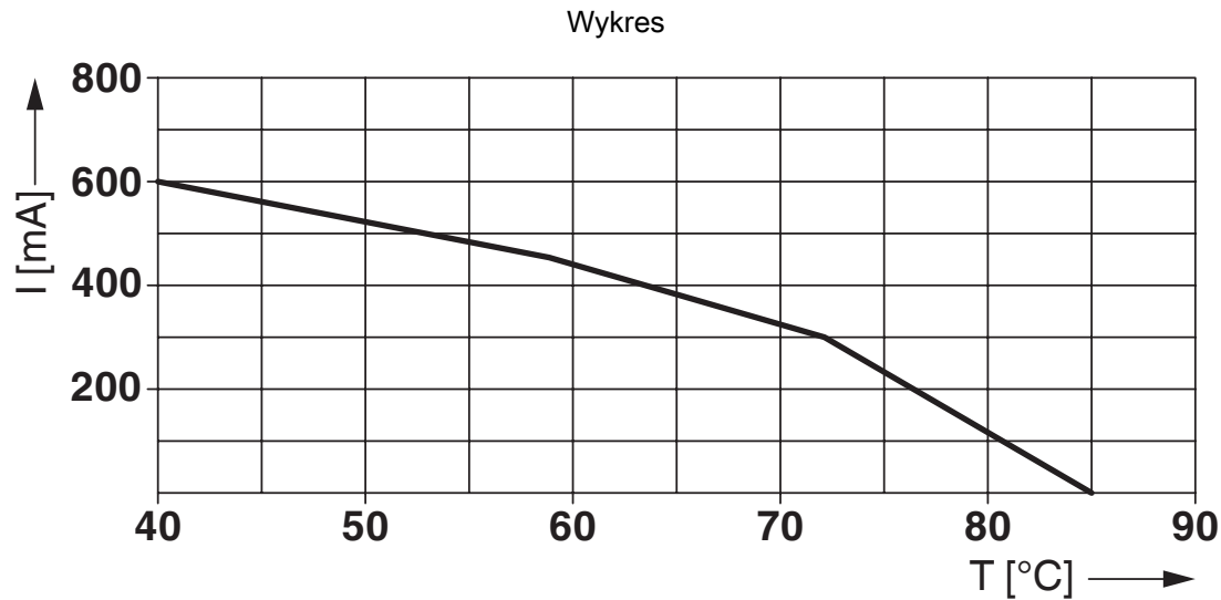
Wykres Derating for Ex-areas (Zone 2, EX ec)
