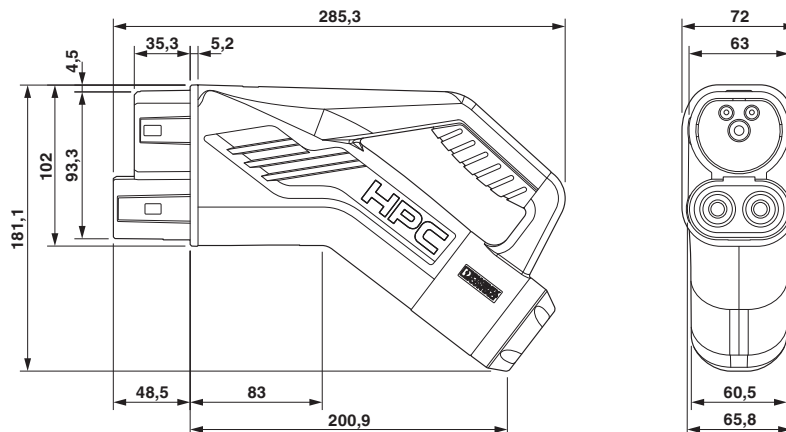
Rysunek wymiarowy
