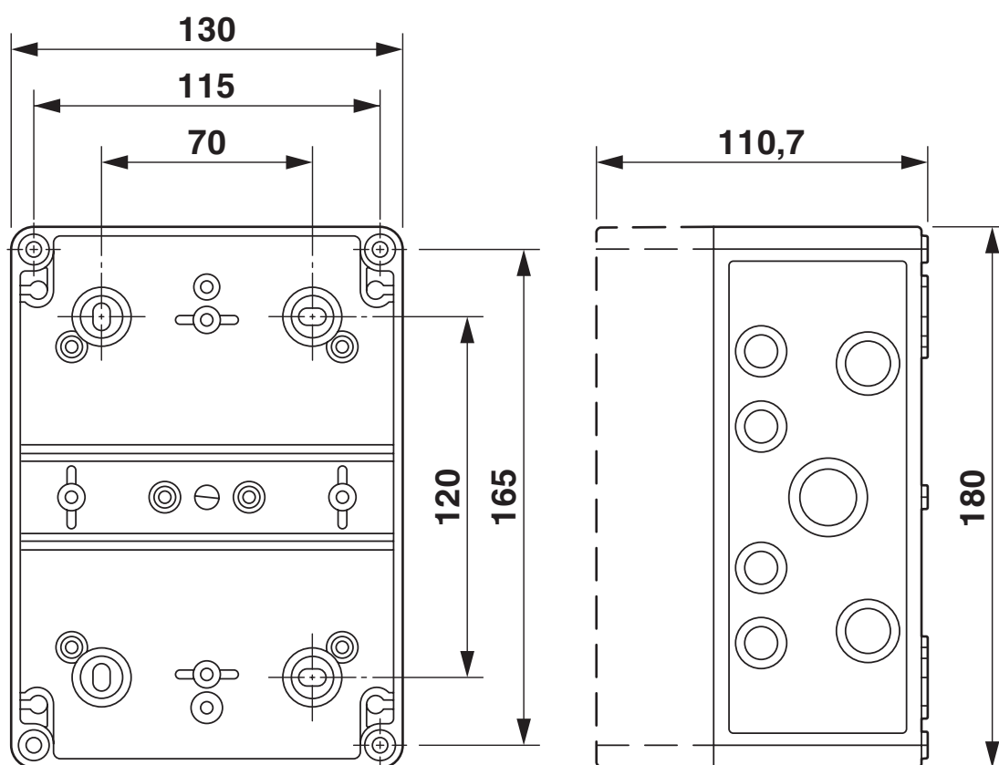
Rysunek wymiarowy
