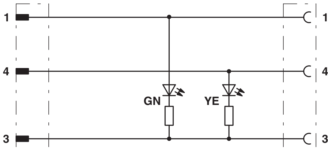
Przyporządkowanie styków wtyków M12 / gniazd M8
