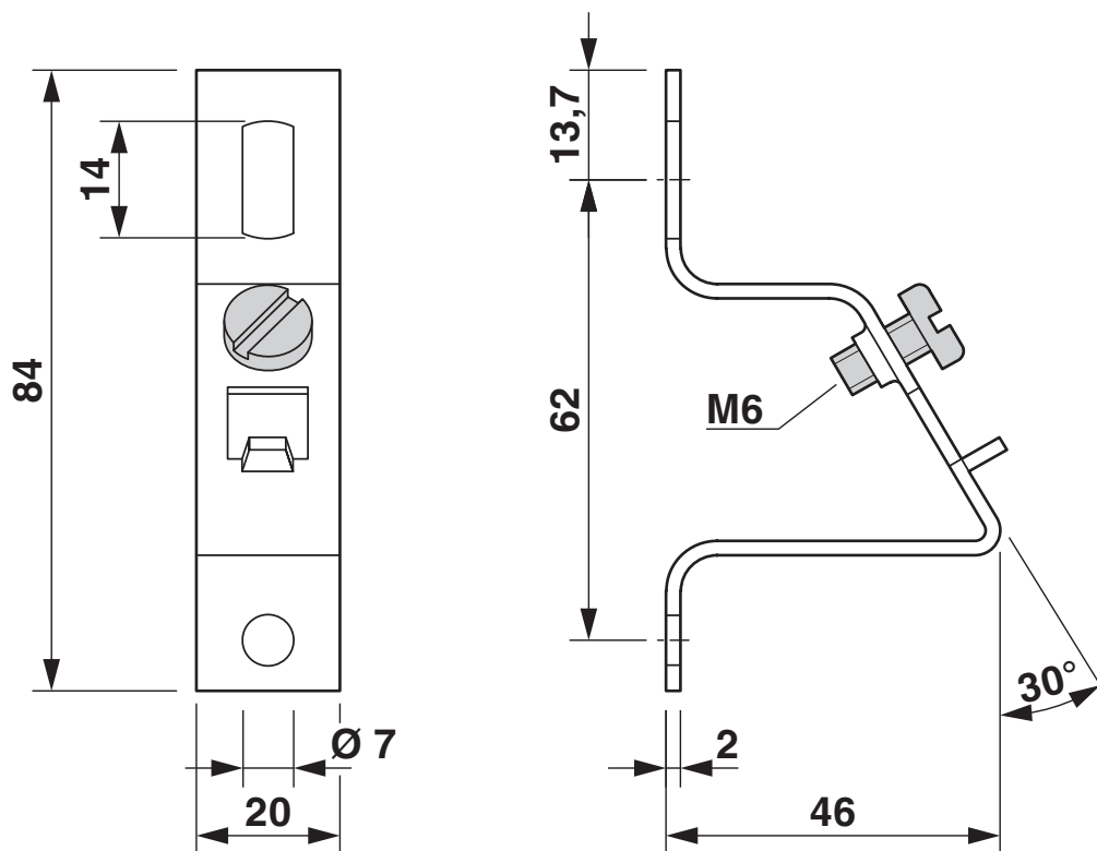
Rysunek wymiarowy
