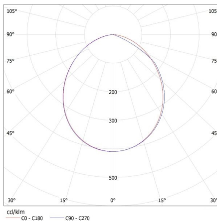
KANLUX S.A. (kat 23550) SEVIA LED 26 / Krzywa rozsyłu światła (biegunowo)
