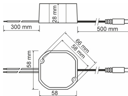
Rys. 1. Widok mechaniczny zasilacza.
