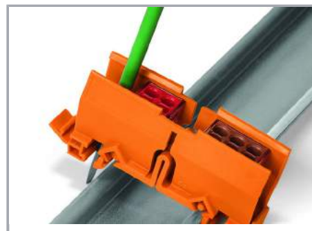
Demontaż adaptera montażowego z szyny TS 35
