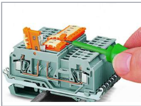
Uchylny łącznik nożowy sygnalizuje stan połączenia i zostaje zakleszczony w krańcowych pozycjach „ON” <-> „OFF”.
