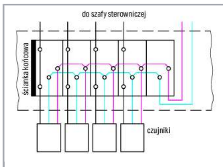
Zasilanie od strony czujników
