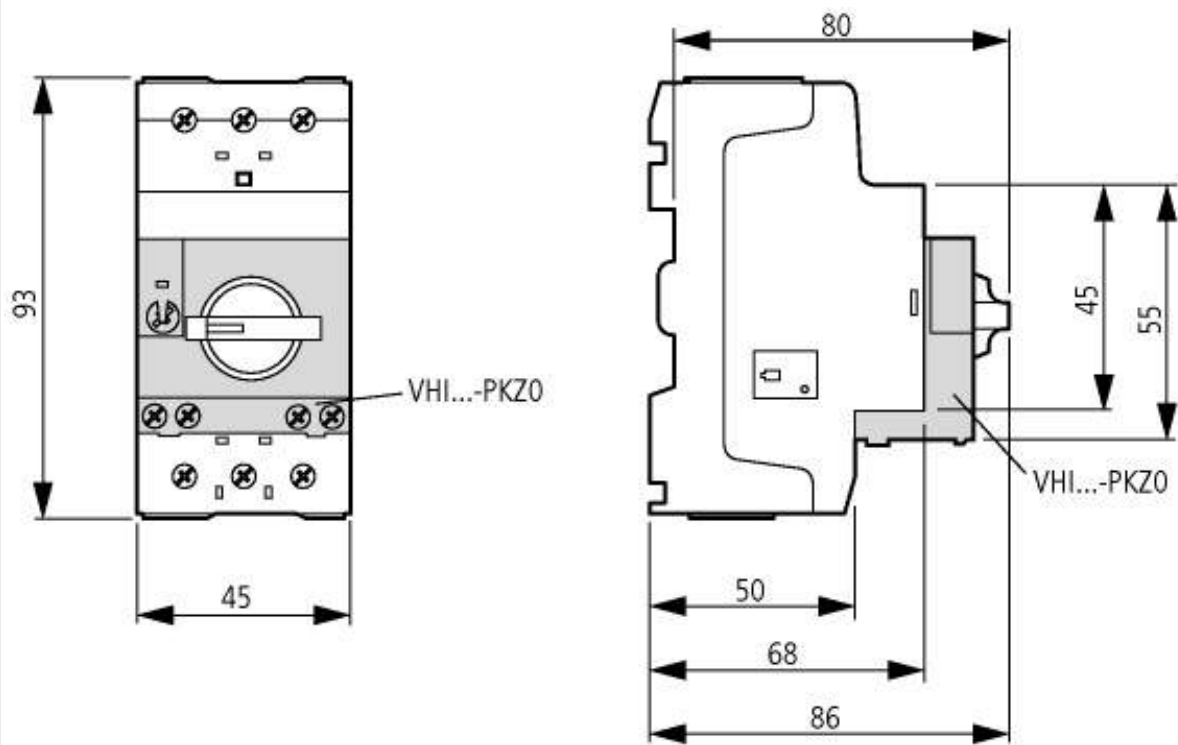
Wyłączniki silnikowe z wyrzadzającym wyłącznikiem pomocniczym PKZM0-...+VHI-...-PKZO
